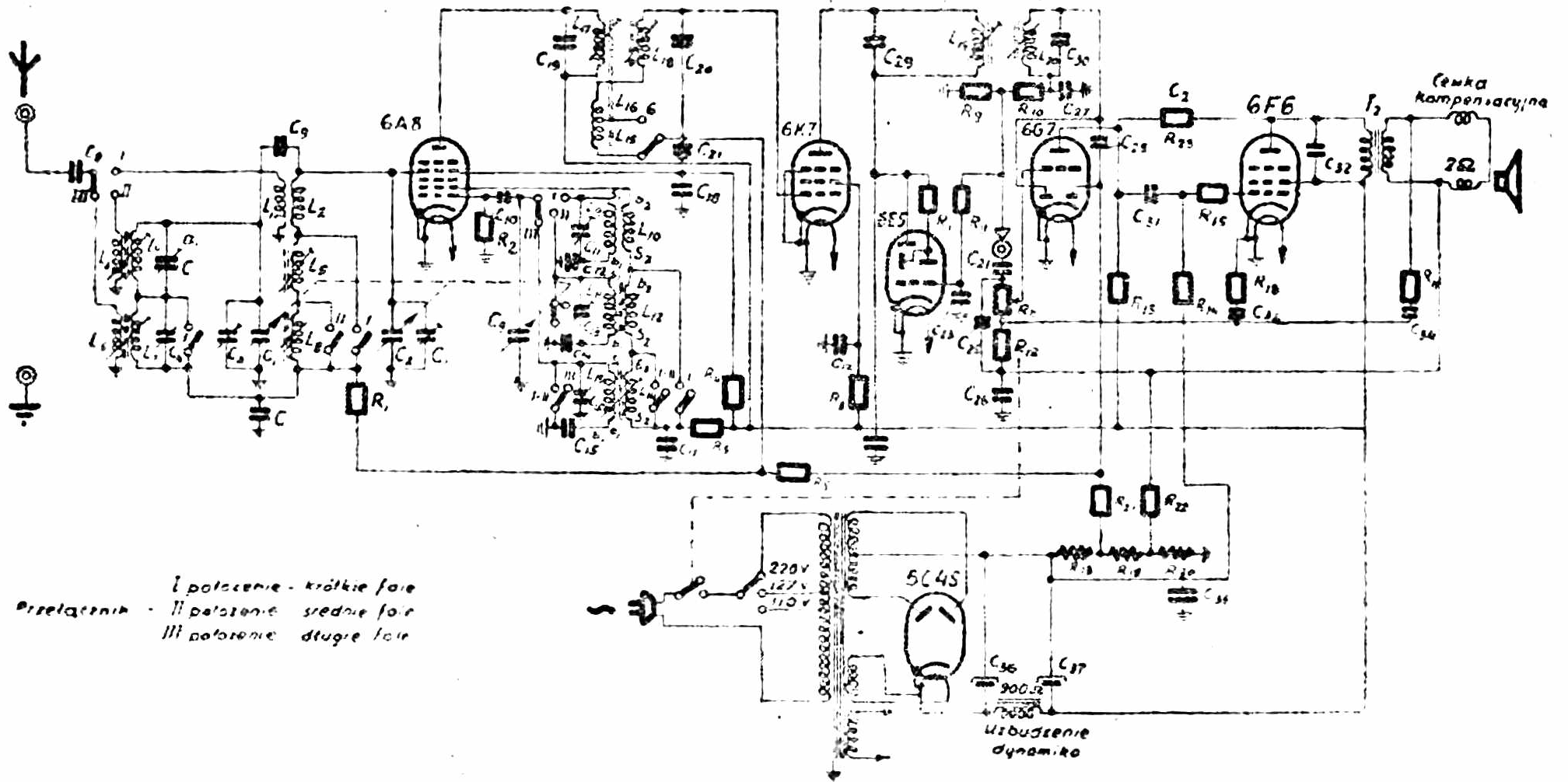
Schemat odbiornika Wefsuper M-557
