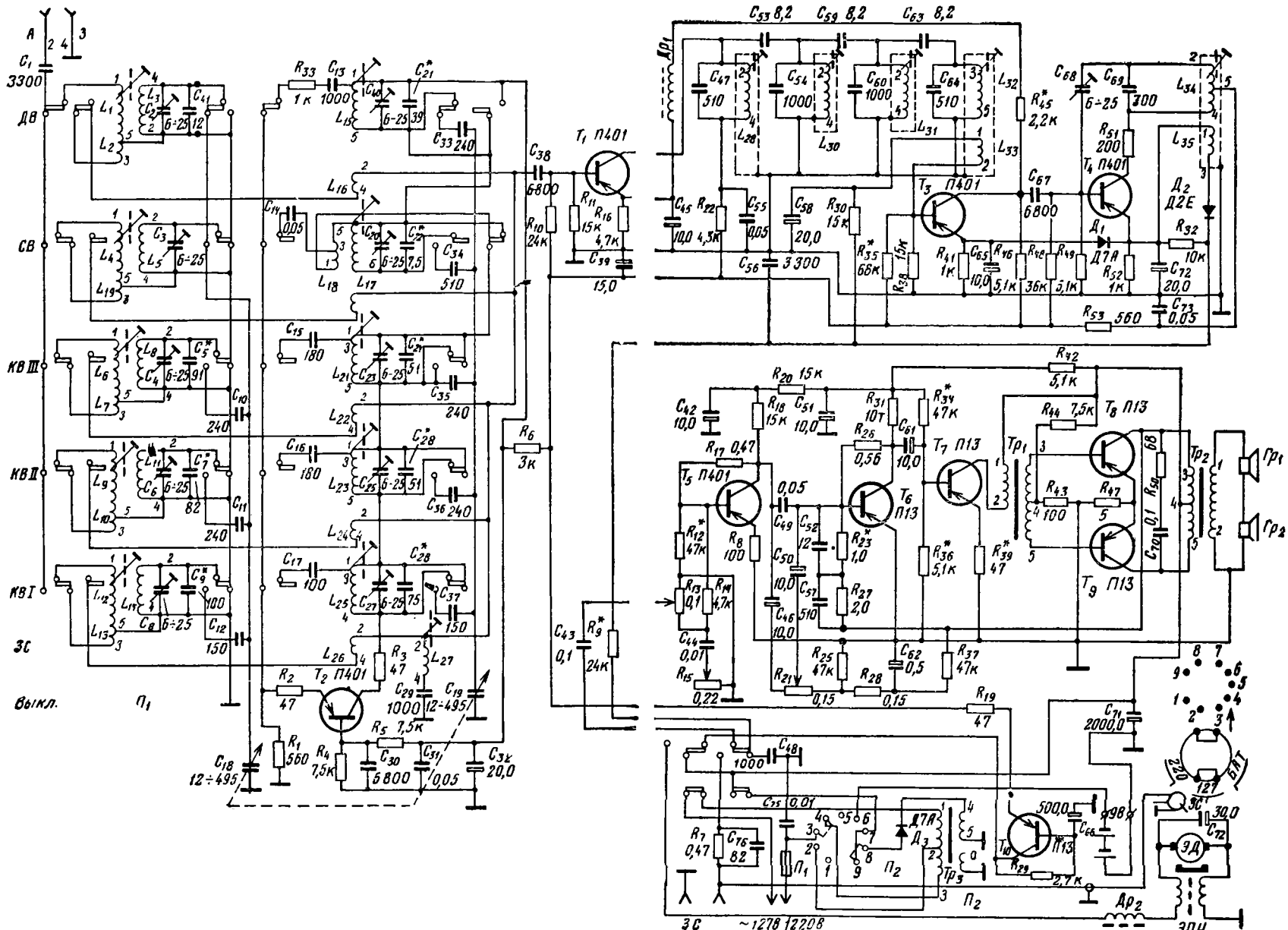
Принципиальные схемы приемника «Родина 60М1» и радиолы «Эфир»
