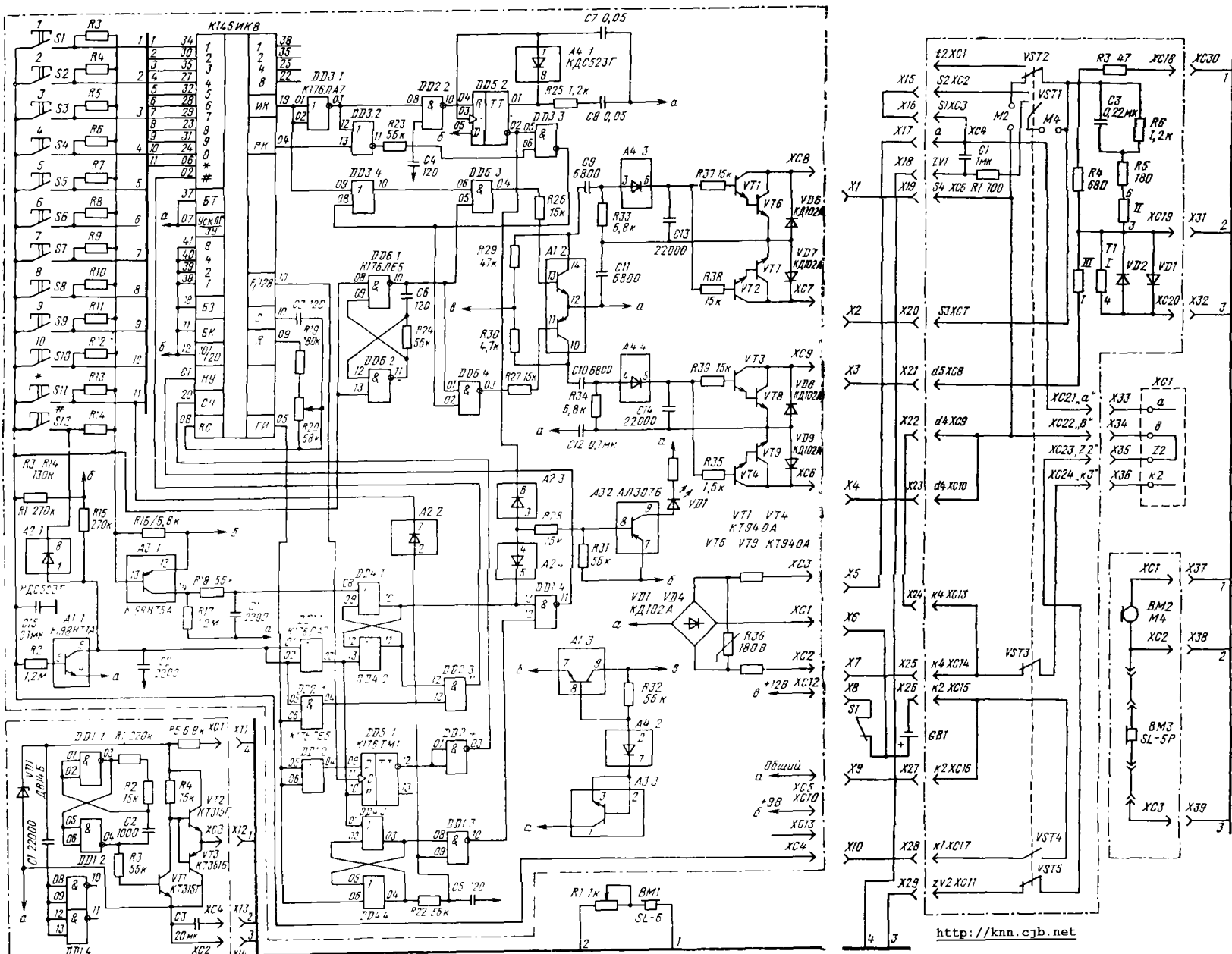
Принципиальная схема телефонного аппарата «Электроника Элетап-микро» (модель 3)
