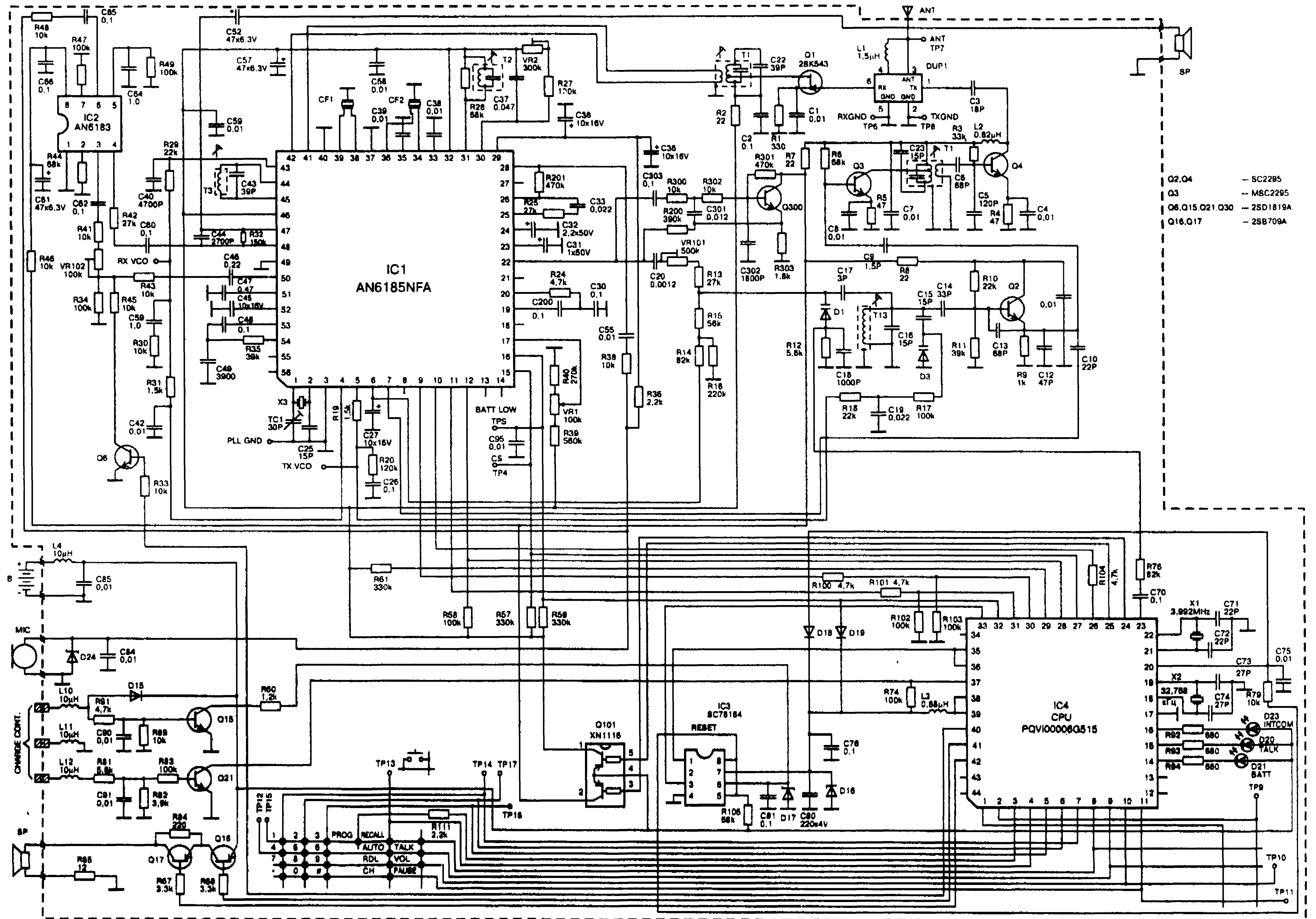
Рис. 2.29. Принципиальная схема носимого блока радиотелефона KX-T4046
