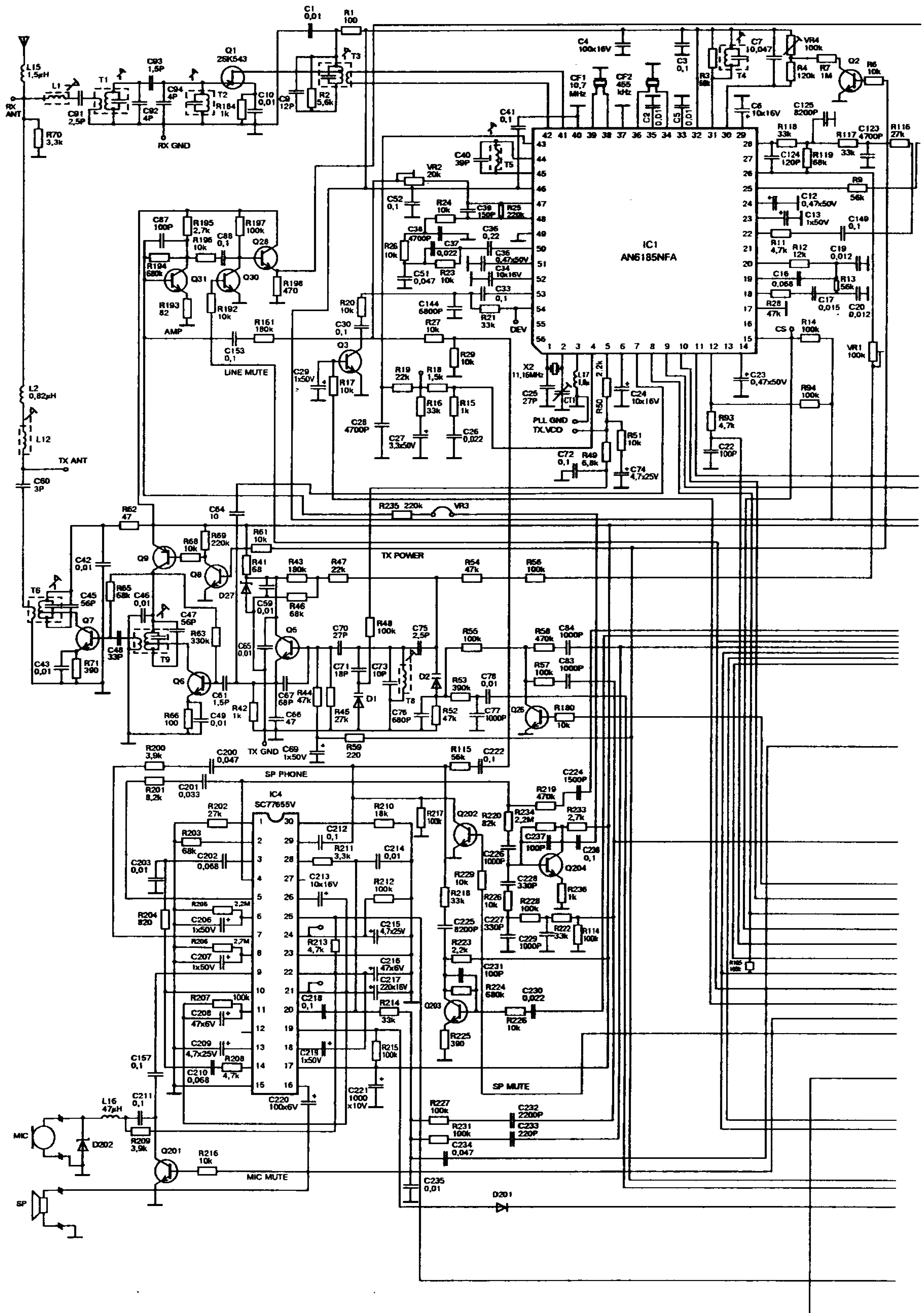
Принципиальная схема базового блока
