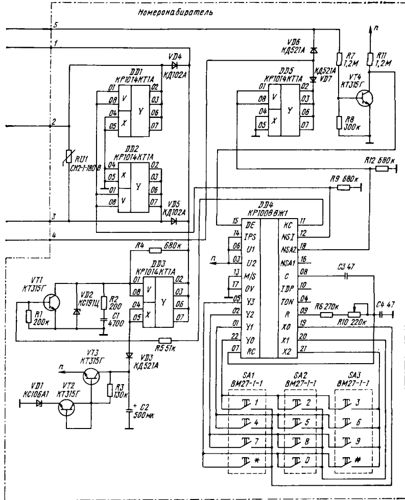
Принципиальная схема телефонного аппарата «Электроника ТА-5-01»
