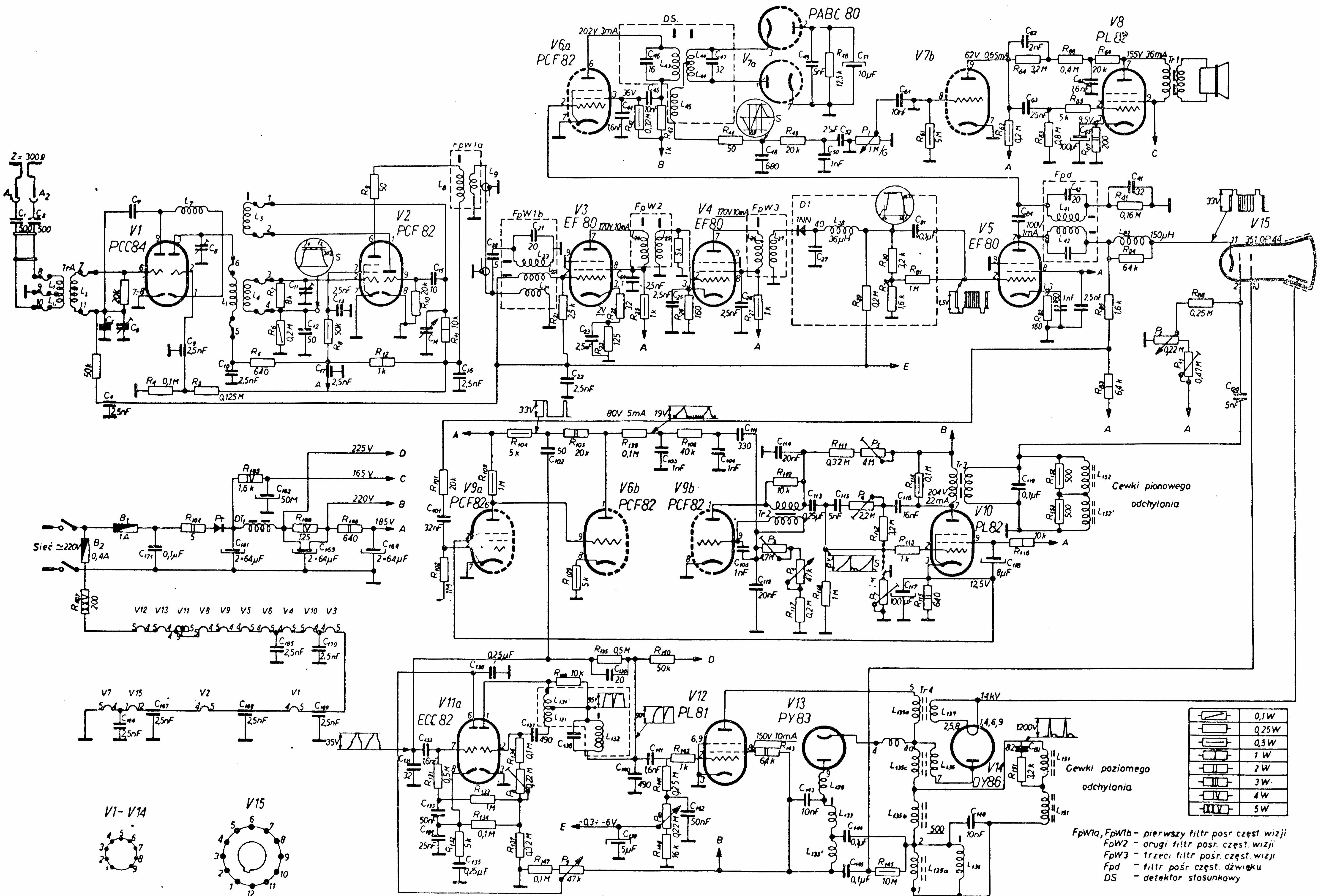
Schemat ideowy odbiornika telewizyjnego Tesla 4102U (Manes) oraz Tesla 4103U (Aleš).
